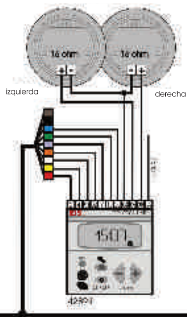
HABITACIÓN CON SINTONIZADOR FM
