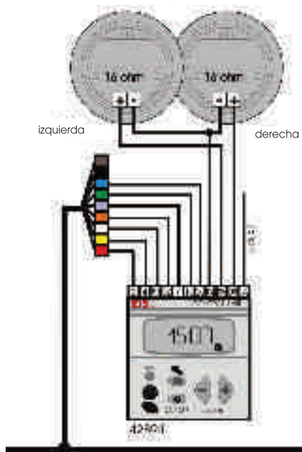
HABITACIÓN CON SINTONIZADOR FM
