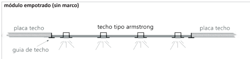
módulo empotrado (sin marco)
